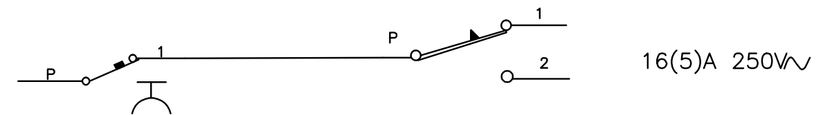
SCHEMA ELETTRICO ELECTRICAL DIAGRAM
